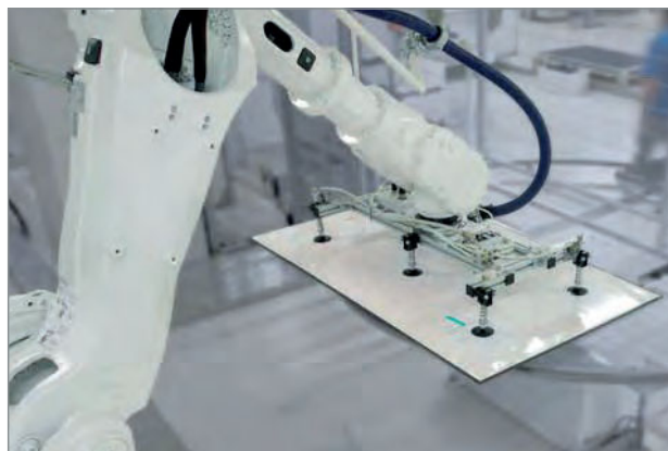
扁平真空吸盘PFTN搬运加工完成的塑料板材
